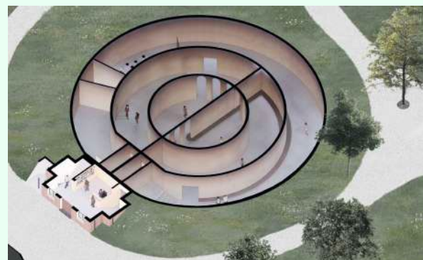
Render doorsnede ondergrondse tentoonstellingsruimte en (linksonder) het receptie- en entreegebied van RADIUS. Beeld door DP6 Architectuurstudio.
